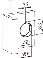
Шаблон для сверления отверстий для установки
