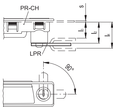
Варианты установки ручки PR-CH
