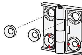
Принцип действия (тип BJ)
